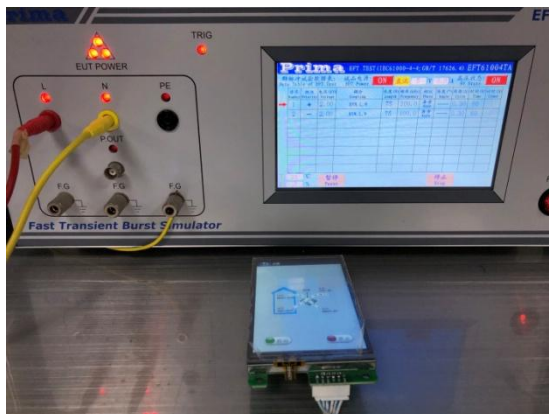
图 4-3 EFT 测试图
