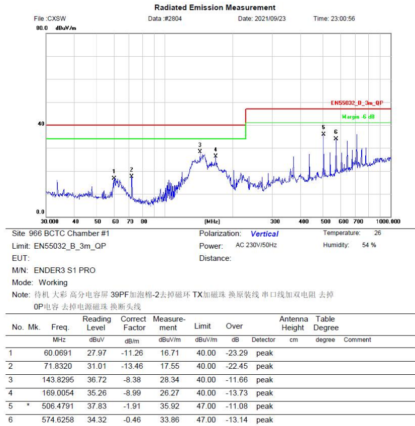
图 4-6 RE 测试垂直方向
