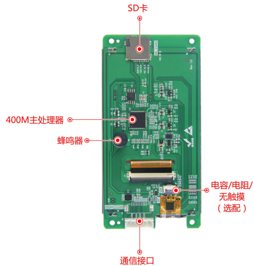
图 1-4 硬件配置图
