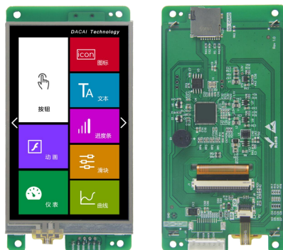
图 1-2 4.3 寸电阻触摸参考图
