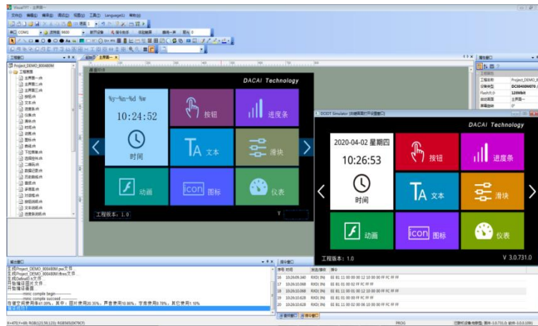
图 5-1 VisualTFT 主界面
