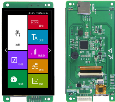
图 1-1 4.3 寸电容触摸参考图
