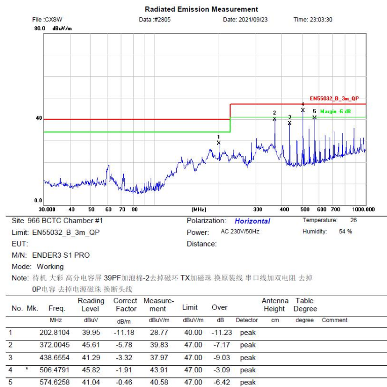
图 4-5 RE 测试水平方向
